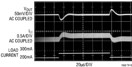
3.3V 到 5V 瞬态响应
