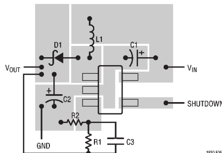
图 6：建议采用的布局
