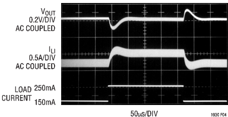
图 4：图 1 所示的升压转换器在带有 10pF 相位超前电容器时的瞬态响应
