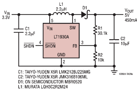
3.3V 到 5V，450mA 升压型转换器
