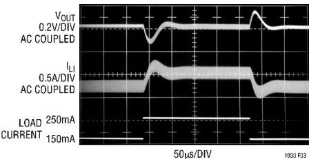
图 3：图 1 所示的升压转换器在没有相位超前电容器时的瞬态响应
