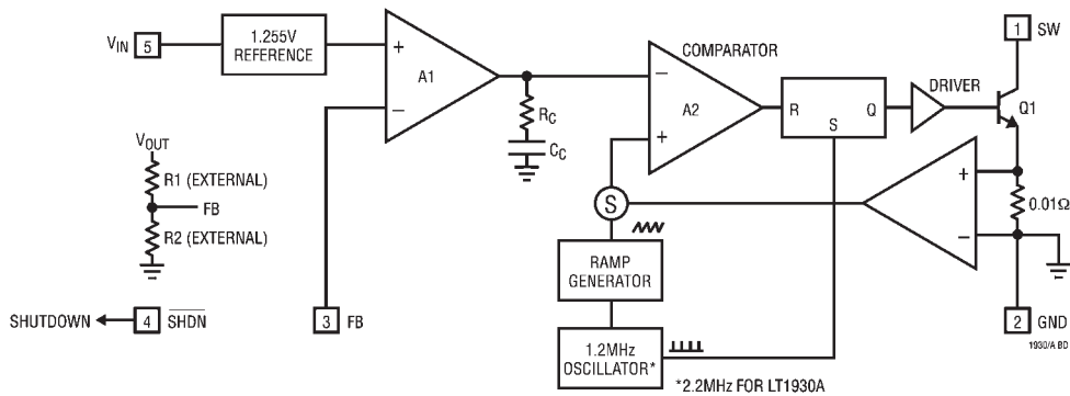
图 2：方框图
