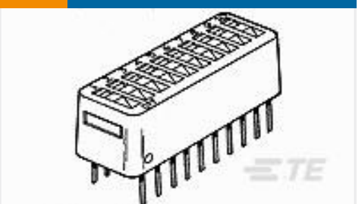
TE 产品编号3-435668-0 DIP SW 10 POSN W/TAPE AU
