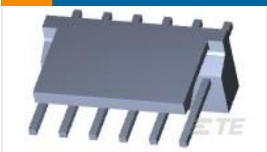
TE 产品编号3-647296-6 06P MTA100 HI-TEMP HDR 15AU TL
