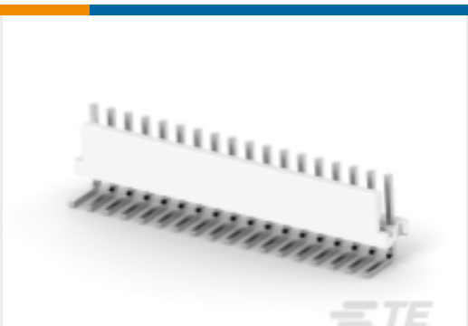
TE 产品编号 4-644755-8 18P MTA156 HDR ASSY SQ RARB F/L
