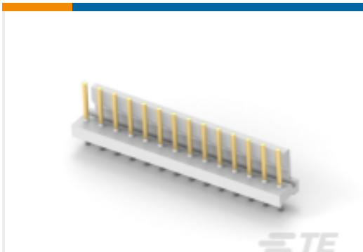
TE 产品编号 4-641209-4 14P MTA156 HDR ASSY FL ST LF
