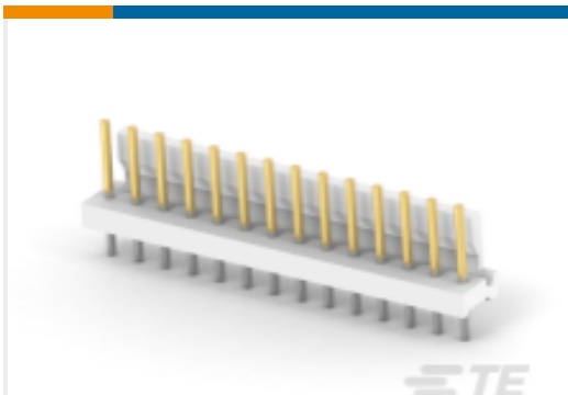
TE 产品编号 4-644760-4 14P MTA156 HDR ASSY FL ST LF
