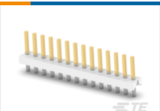
TE 产品编号 4-644756-4 14P MTA156 HDR ASSY STR AU LF
