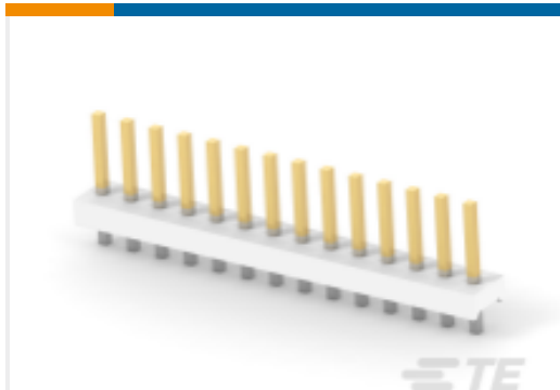
TE 产品编号 4-641203-4 14P MTA156 HDR ASSY PL 30AU LF
