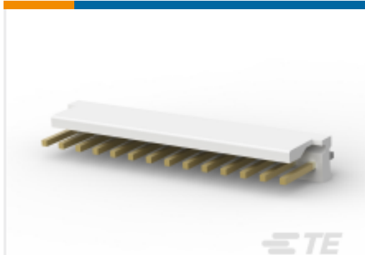
TE 产品编号 4-641208-4 14P MTA156 HDR ASSY FL ST LF
