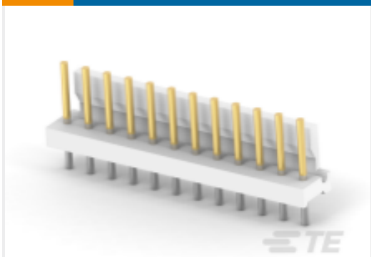
TE 产品编号 4-644760-2 12P MTA156 HDR ASSY FL ST LF
