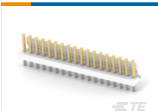
TE 产品编号 4-641210-8 18P MTA156 HDR FLRA FB 30AU LF
