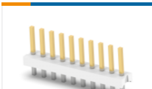
TE 产品编号 4-644756-0 10P MTA156 HDR ASSY STR AU LF
