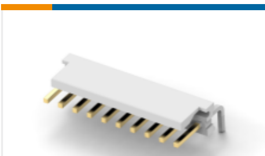
TE 产品编号 4-644761-0 10P MTA156 HDR ASSY R/A F/L LF
