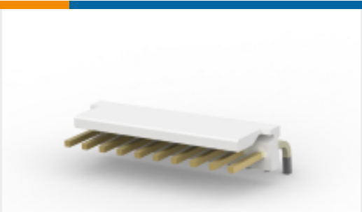
TE 产品编号 4-641210-0 10P MTA156 HDR FLRA FB 30AU LF
