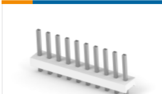
TE 产品编号 4-641202-0 10P MTA156 HDR ASSY PL 30AU LF
