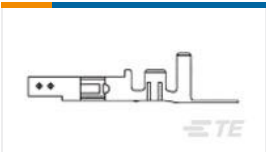
TE 产品编号1586841-4 VAL-U-LOK SKT 16AWG PHBZAU LP
