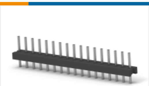
TE 产品编号 1-644750-7 17P MTA156 HDR ASSY STR RND SN
