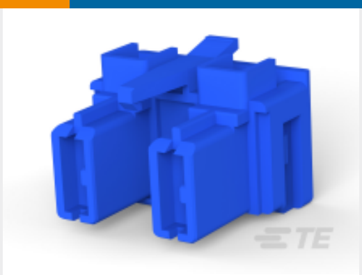
TE 产品编号1-1743165-8 PL EX 2P .250 (6.3 MM) FLAG BLUE
