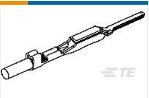
TE 产品编号1376039-4 040 NK TAB CONT PRE TIN
