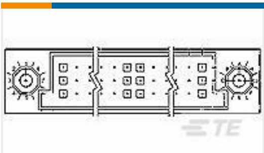
TE 产品编号1-532447-2 HDI PIN ASSY 3 ROW 225 POS
