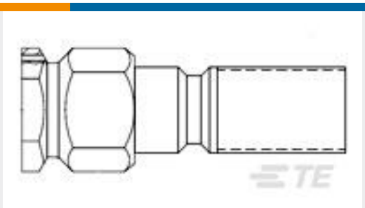
TE 产品编号1051785-1 SMA CABLE PLUG 2031 8028 92
