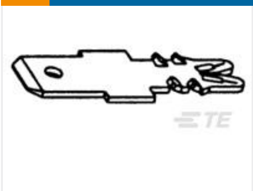
TE 产品编号3-1601174-2 .187 X .032 TAB STD SIAMEZE
