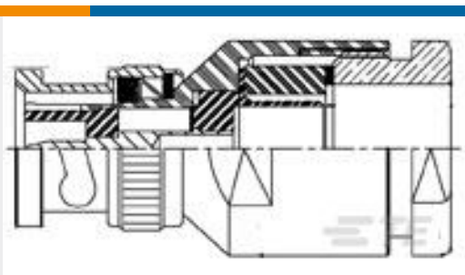
TE 产品编号1-1478404-0 BNC Str Plg PS 75Ohm Silver RG59B /U, 62A
