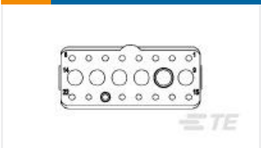
TE 产品编号1738154-1 Insert Asy,Skt,Arr 22,Environ,Key B
