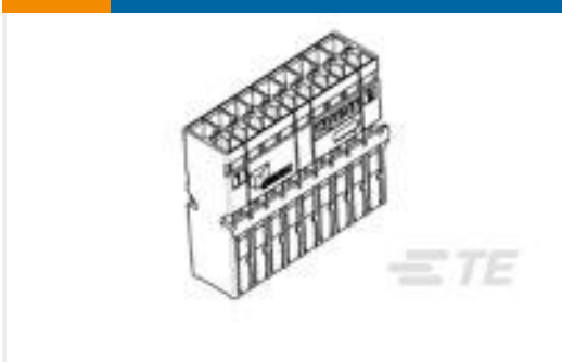
TE 产品编号1456867-3 PLG ASSY,2X8,UNSEALD, 0.64,Gen
