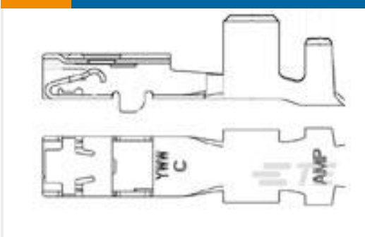
TE 产品编号1326030-3 2.8MM RECP,UNSEAL,14-16AWG
