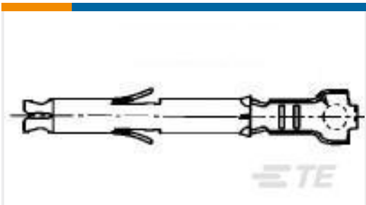
TE 产品编号170366-1 MINI UNIVERSAL M-N-L SOCKET LP
