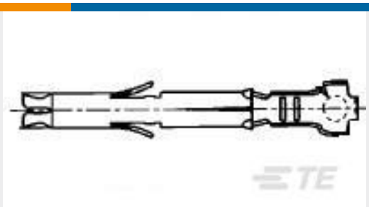
TE 产品编号170365-1 MINI UNIVERSAL M-N-L SOCKET LP
