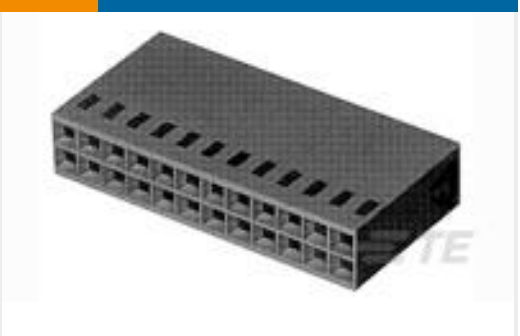
TE 产品编号1-87456-2 16 MODIV HSG DR MRKD .100CL
