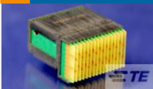
TE 产品编号1410303-1 MULTIGIG RT2 7RW DC RTM
