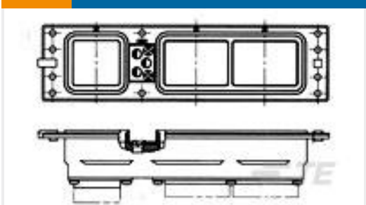
TE 产品编号1996164-1 ARINC 600,SZ 2,RCPT
