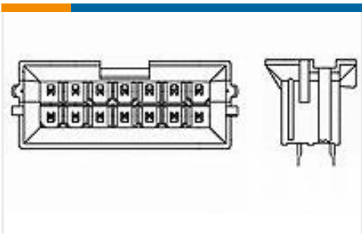
TE 产品编号1-1586585-0 10P VAL-U-LOK BMI VRT HDR V2
