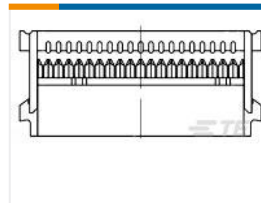
TE 产品编号3-1437021-4 609-3441=FSKT IDC S 34 30AU PL
