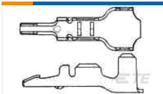
TE 产品编号170197-1 MINI AMP-IN 24-20 AWG
