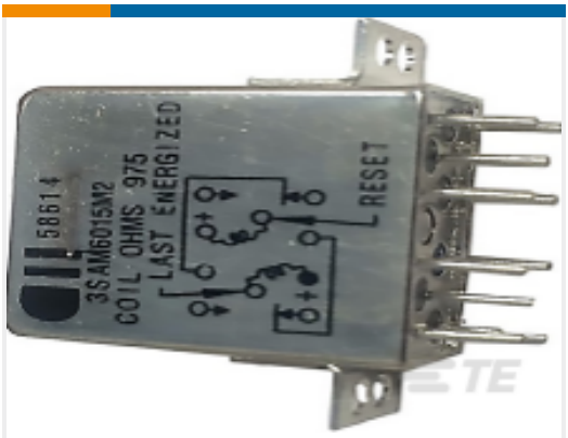
TE 产品编号 1-1617088-4 3SAM1820A2 = M39016/32-002
