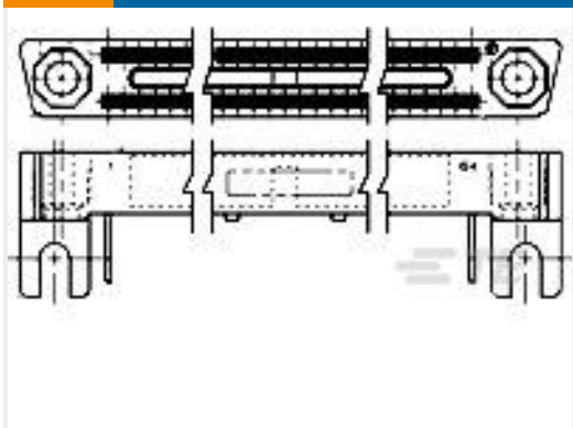
TE 产品编号1-445185-0 MINI BOX RCPT ASSY/MTG EARS
