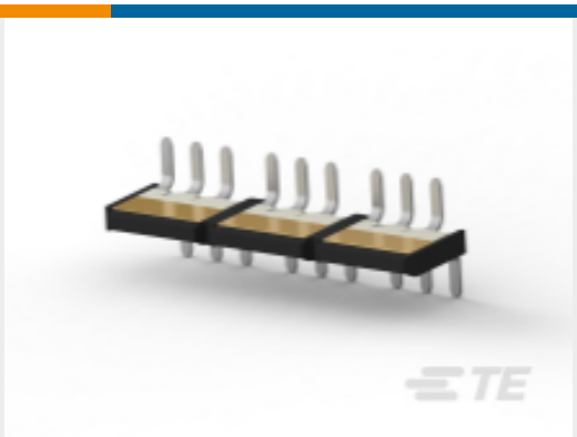
TE 产品编号2085196-1 Connector Blade MC-P3S0 Mini Crown Edge
