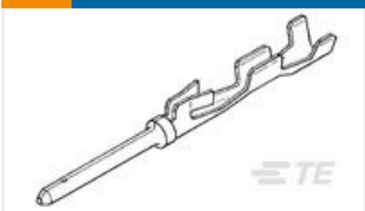
TE 产品编号1-745267-0 CONT,PIN,HDE,#18-22
