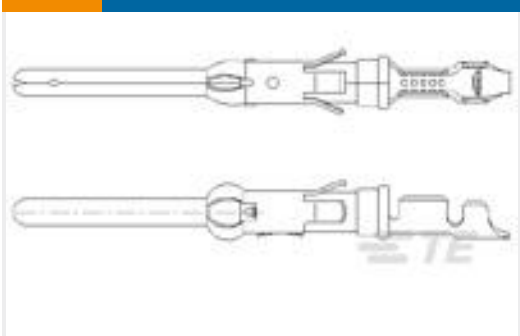
TE 产品编号163085-1 .062 DIA PIN ASS 3+
