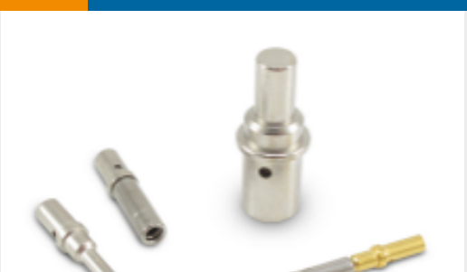
TE 产品编号0462-201-20141 DEUTSCH 实芯端子
