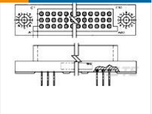
TE 产品编号443857-2 3 ROW BOX RECEPTACLE
