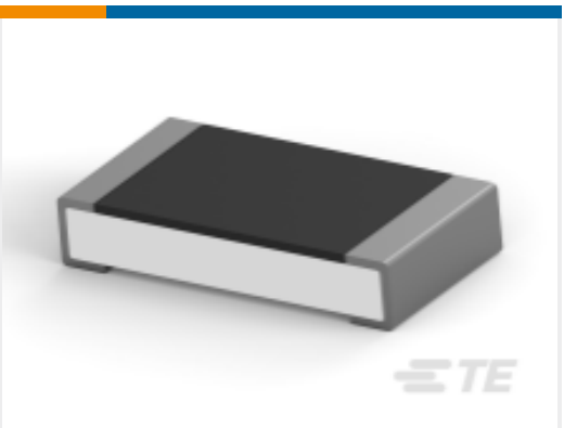
TE 产品编号1-2176388-6 RQ 1206 14R3 0.1% 10PPM 5K RL
