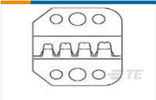
TE 产品编号90574-2 PROCRIMPER DIE ASSY COMM MNL
