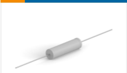
TE 产品编号8-2176414-6 7W STD M/OX 5% 68K
