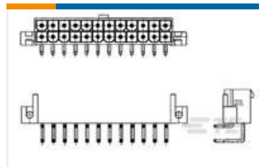
TE 产品编号1-1586043-2 12P VAL-U-LOK R/A HDR SCRMT V2
