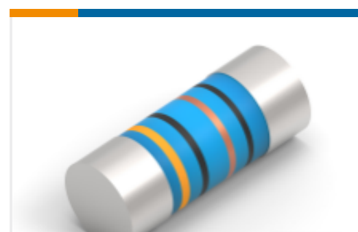
TE 产品编号1-2176316-5 MELF SMA_A 1K5 0.1% 15PPM 0207 1W
