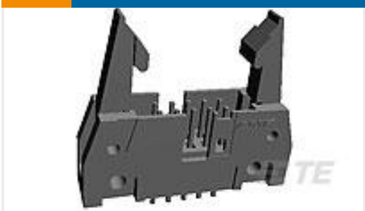
TE 产品编号1-5102321-0 A/L UNIV HDR 50P VERT LG LAT
