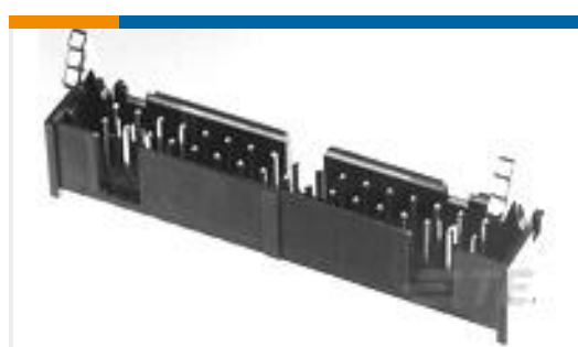
TE 产品编号2-1761608-8 IDC LOW PRO HDR 24P VERT SHT L
