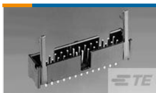
TE 产品编号104315-7 040 LOPRO HDR RA 30DP LATCH
