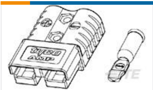
TE 产品编号1446000-2 120A PWR PROD KIT,6 AWG,BLUE
