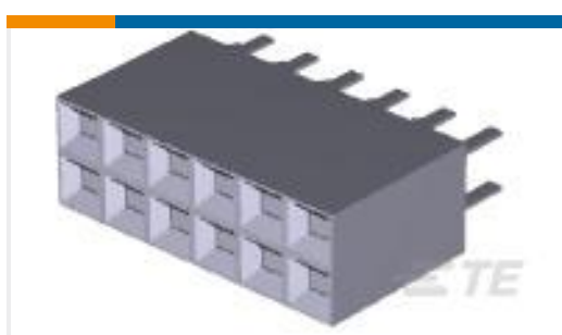
TE 产品编号534206-6 12 MODII VRT DR CE 100/115
