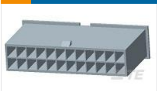
TE 产品编号1-1969612-0 10P FH PLUG VAL-U-LOK V0
