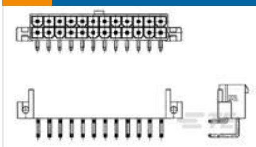
TE 产品编号1-1586043-0 10P VAL-U-LOK R/A HDR SCRMT V2
