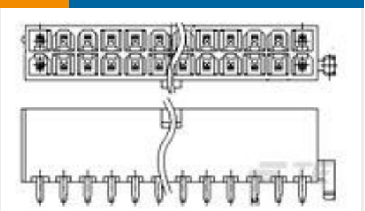
TE 产品编号2-1734774-1 PCI EXP 3.1L 98 POS WHT 30u"
