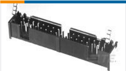
TE 产品编号2-1761606-3 IDC LOW PRO HDR 10P VERT LG LAT BLUE
