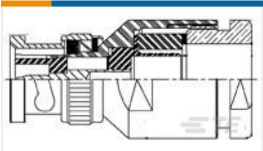
TE 产品编号1-1478402-0 BNC Str Plg PS 50Ohm Silver RG174A /U, 18
