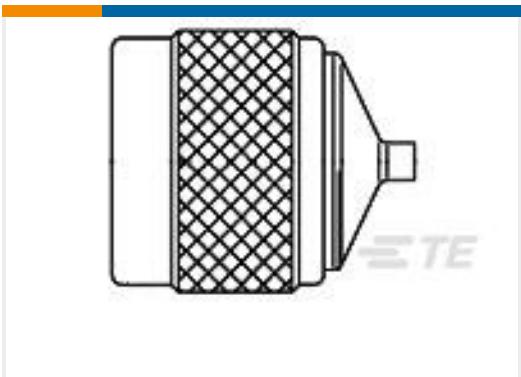
TE 产品编号1046234-1 SCD,1250 1119 00,N
