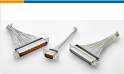
TE 产品编号 204509-8 AMPLIMITE,ASY,PLUG,90,5
