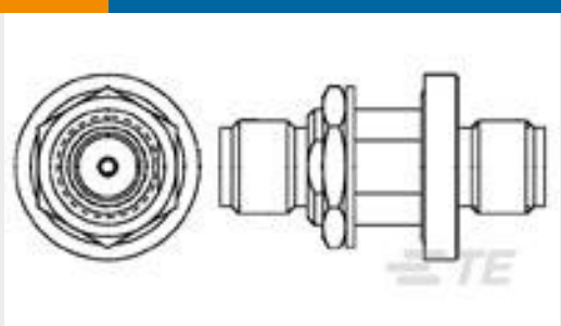
TE 产品编号1054874-1 2084 1100 00
