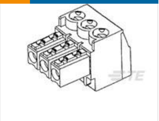
TE 产品编号284509-3 3P TERMI-BLOK PLUG STACK 3,8
