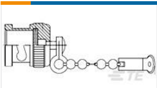
TE 产品编号1-1337524-0 BNC Plg DCap & Chn Nickel Pltd
