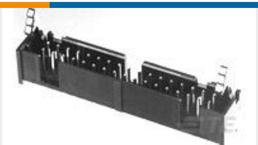
TE 产品编号1-1761608-5 IDC LOW PRO HDR 50P VERT SHT L
