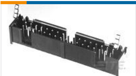
TE 产品编号1-1761608-1 IDC LOW PRO HDR 34P VERT SHT L
