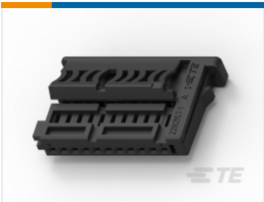
TE 产品编号2282157-1 11POS,NANOMQS,REC HSG,CODA
